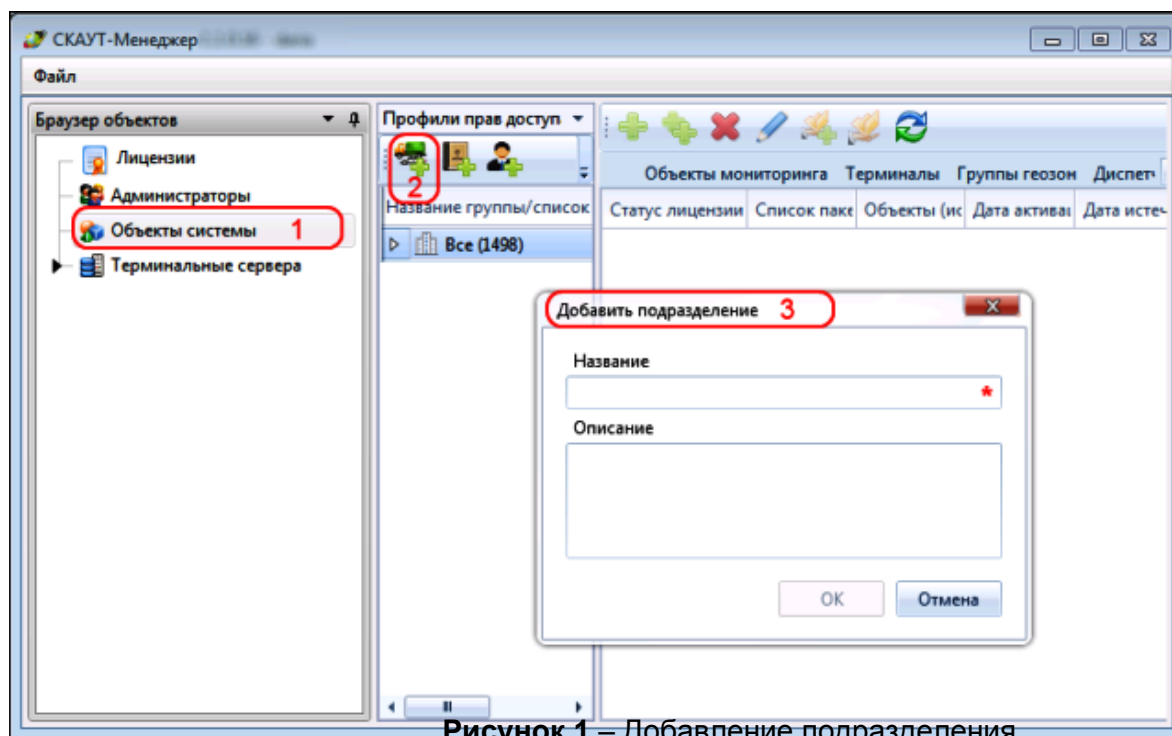
Рисунок 1 – Добавление подразделения
